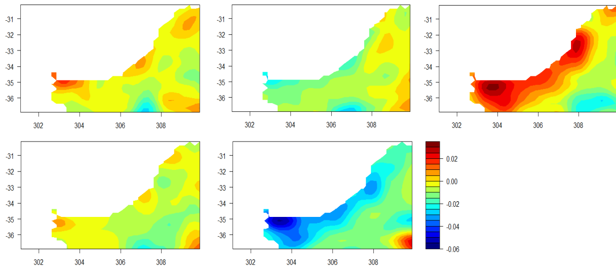
Figura 35 – Composite de anomalía de altura de nivel del mar asociados a los WRs de primavera.
