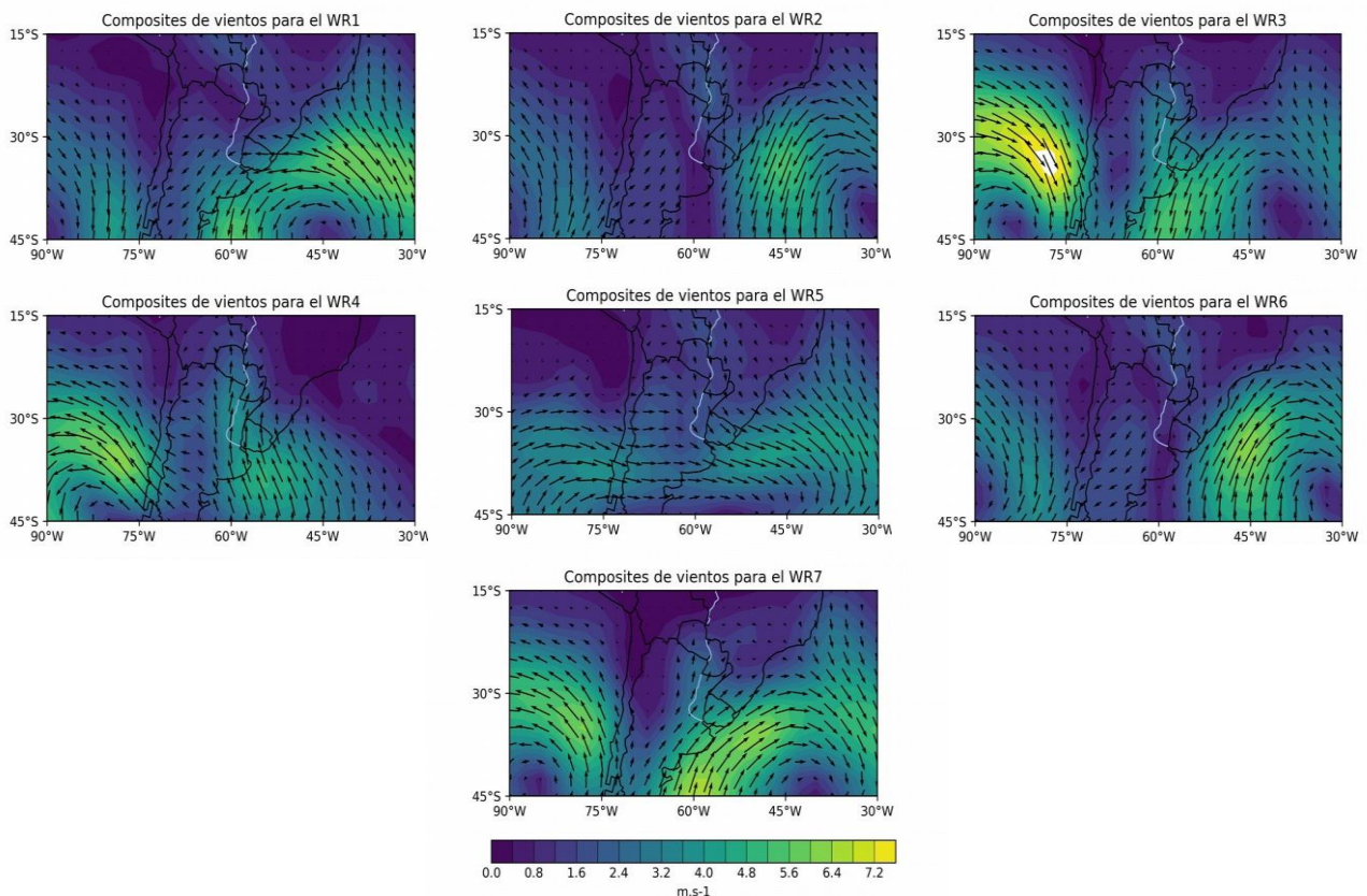
Figura 17 – Regímenes de circulación durante invierno.
